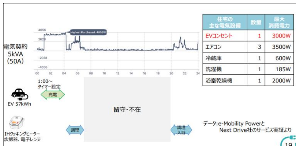
図４－９ 非オール電化家庭におけるEVへの充電状況の一例
