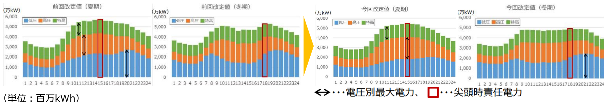
前回改定（現行）と今回申請の需要ロードカーブの比較
